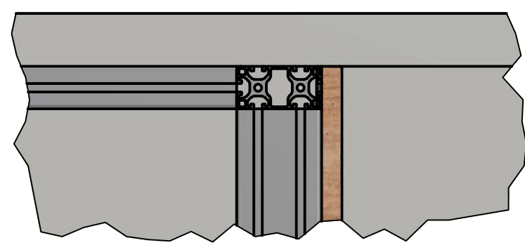
A ( 1 : 5 )
